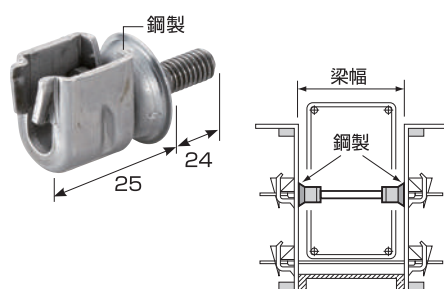
セパレーターB型寸法=梁幅
