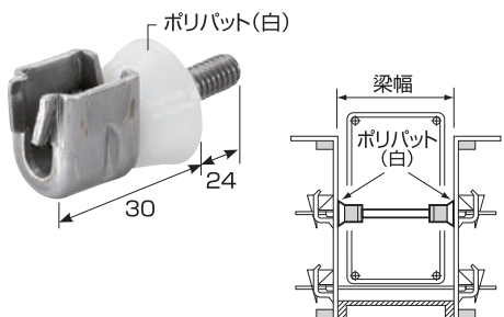
セパレーターB型寸法=梁幅-10mm
