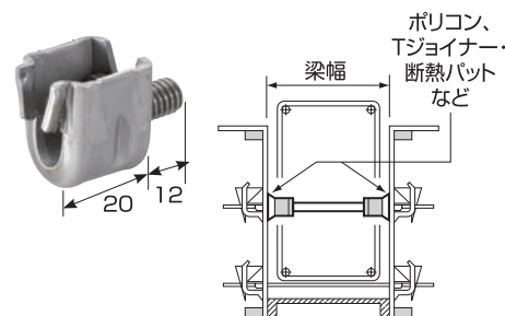
セパレーターB型寸法=梁幅-40mm
