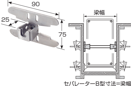
セパレーターB型寸法=梁幅
