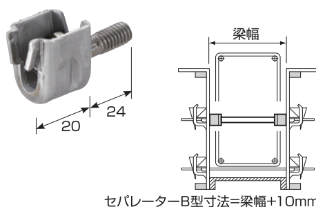
セパレーターB型寸法=梁幅+10mm
